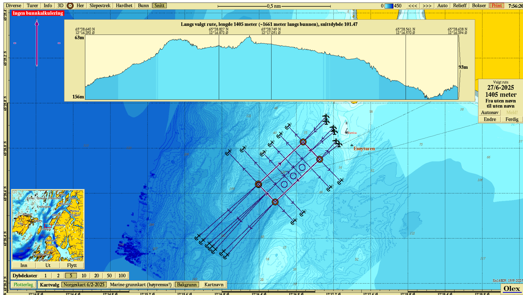
Figur 3.2 Dybdesnitt under planlagt anleggsramme ved den planlagte lokaliteten, Kartet har nordlig orientering.
