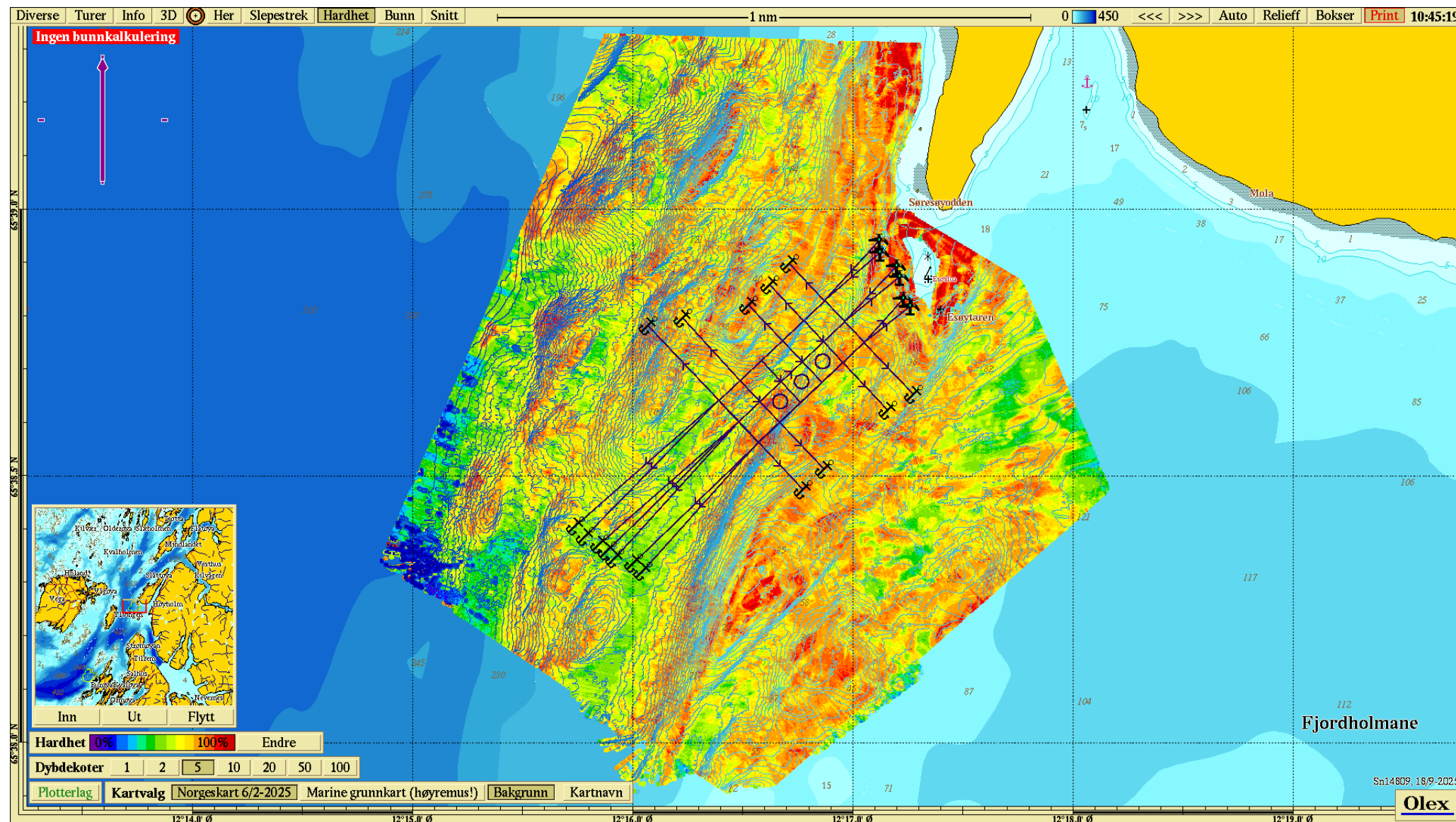
Figur 3.4. Kartlegging av relative sedimenthårdhet. Relativ hardhet er representert ved fargekoder hvor rød farge indikerer 100% hardhet, mens lilla indikerer 0% hardhet. Kartet har nordlig orientering.
