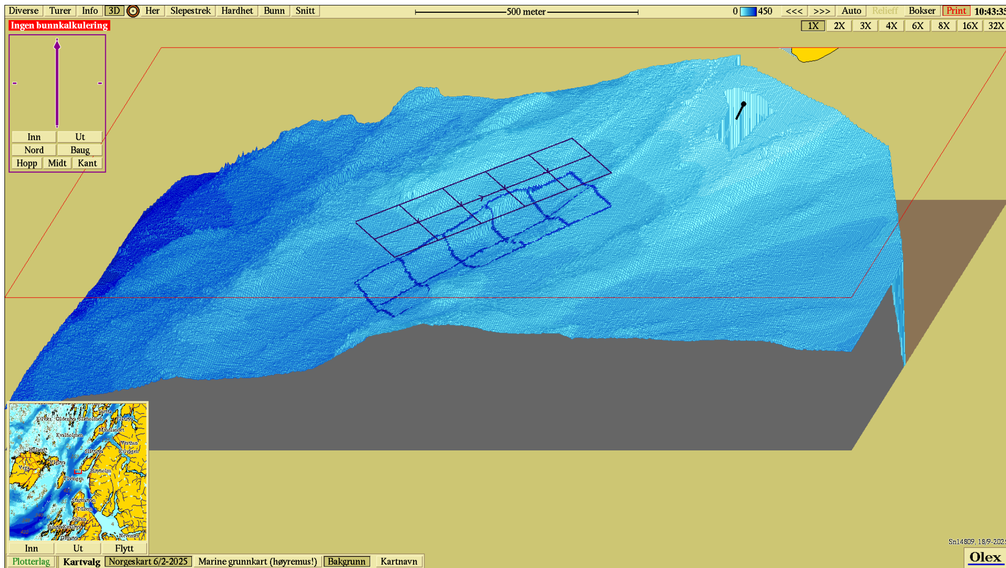
Figur 3.3. Eksempel på 3D visning av oppmålt batymetri. Kartet har nordlig orientering.
